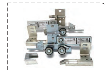
M2Z(T)S8 TKE замок ДШ
