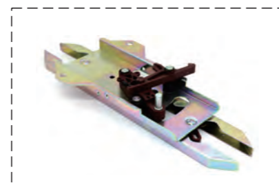
3300AP Fermator schindler отводка ДК
