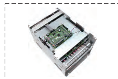
HIVD900G Hyundai Частотник
