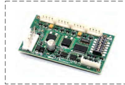
RS14 OTIS PCB основная плата
