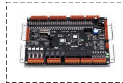
KLS-MCU Cannu основная плата
