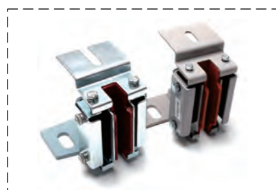
120*10/16mm общий башмак
