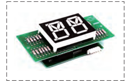
DCI-230 DCI-270 LG Sigma плата дисплея
