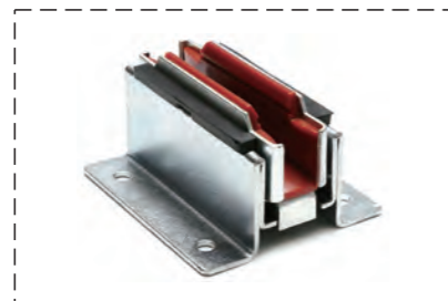
120*10/16mm KONE башмак
