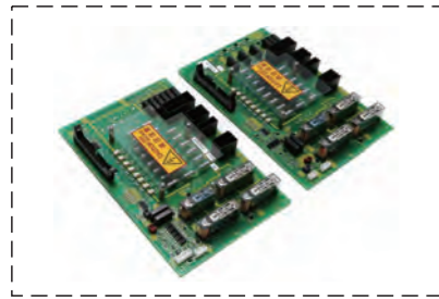
MC24A MC23A Fujites PCB плата
