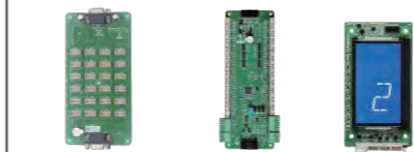
Плата коммуникации управления кабины Плата кабины Плата поста вызова
