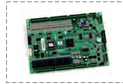
SM-01-F Step основная плата
