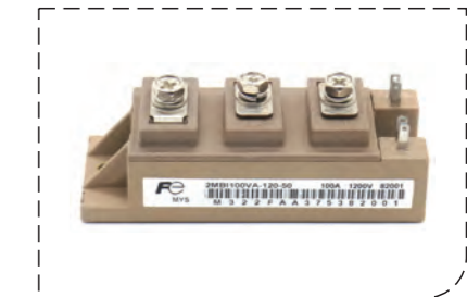
2MBI100VA-120-50 FUJI IGBT модуль
