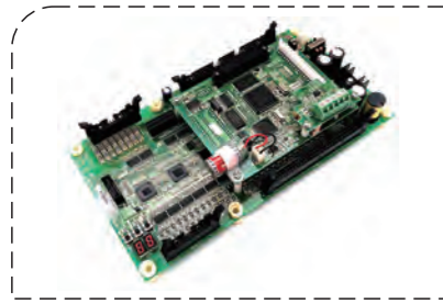
GHE-FMT Hitachi основная плата
