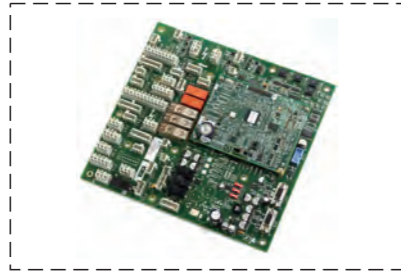
GECB-AP OTIS основная плата
