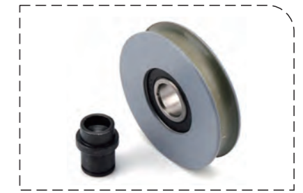
65*13*6202 Hitachi ролик
