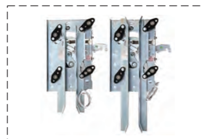
FWL-01 Canny отводка ДК
