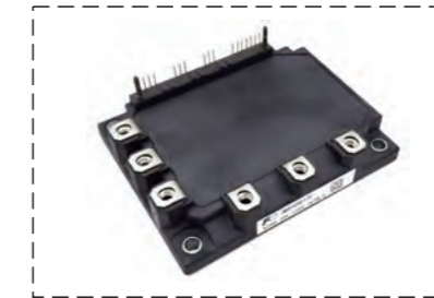
7MBP50RE120 FUJI IGBT модуль
