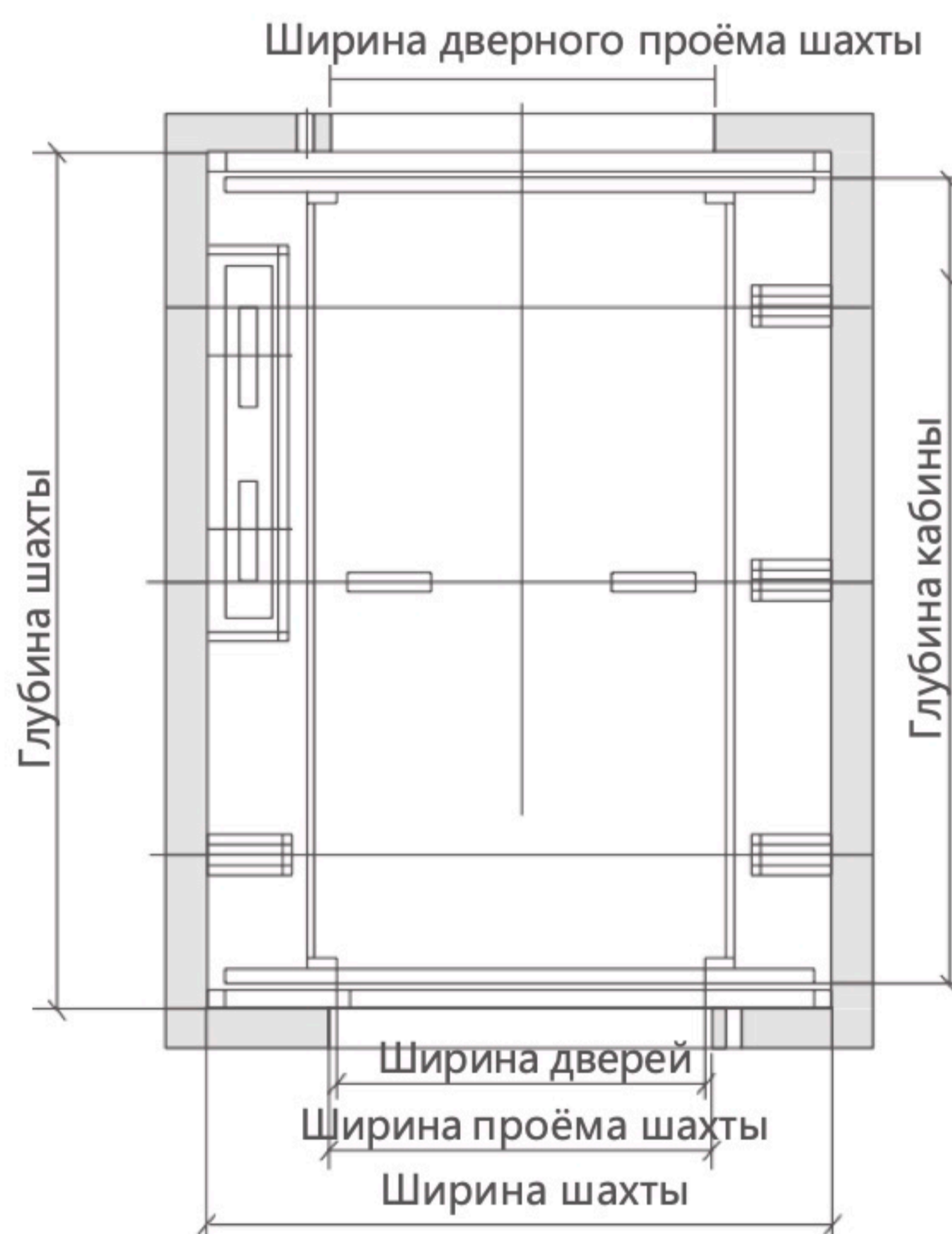
Рисунок макета шахты
