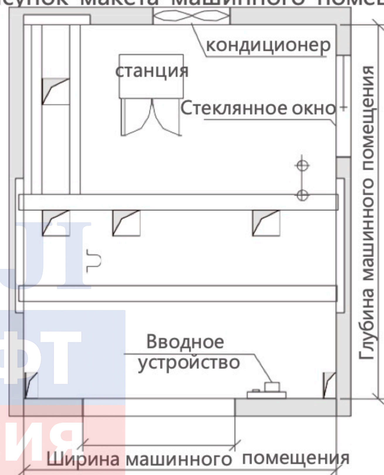
Рисунок макета машинного помещения
